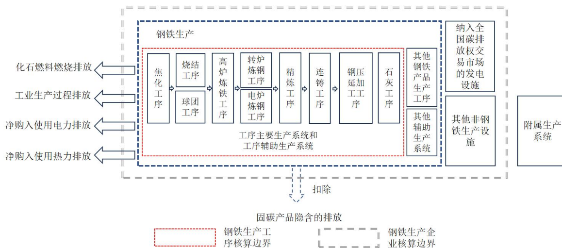
图2 钢铁生产温室气体排放核算边界示意图
